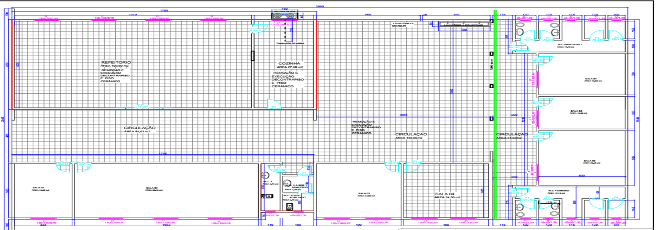
REFORMA GERAL 656,82 M2 ESCALA 1 : 100
